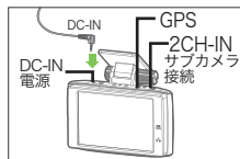
電源ケーブル、GPS、サブカメラ接続ケーブルを配線
